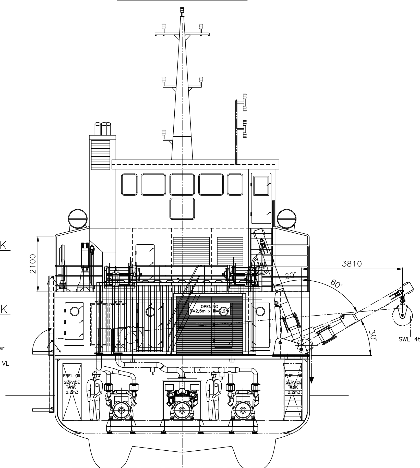
SECTION FR.17
