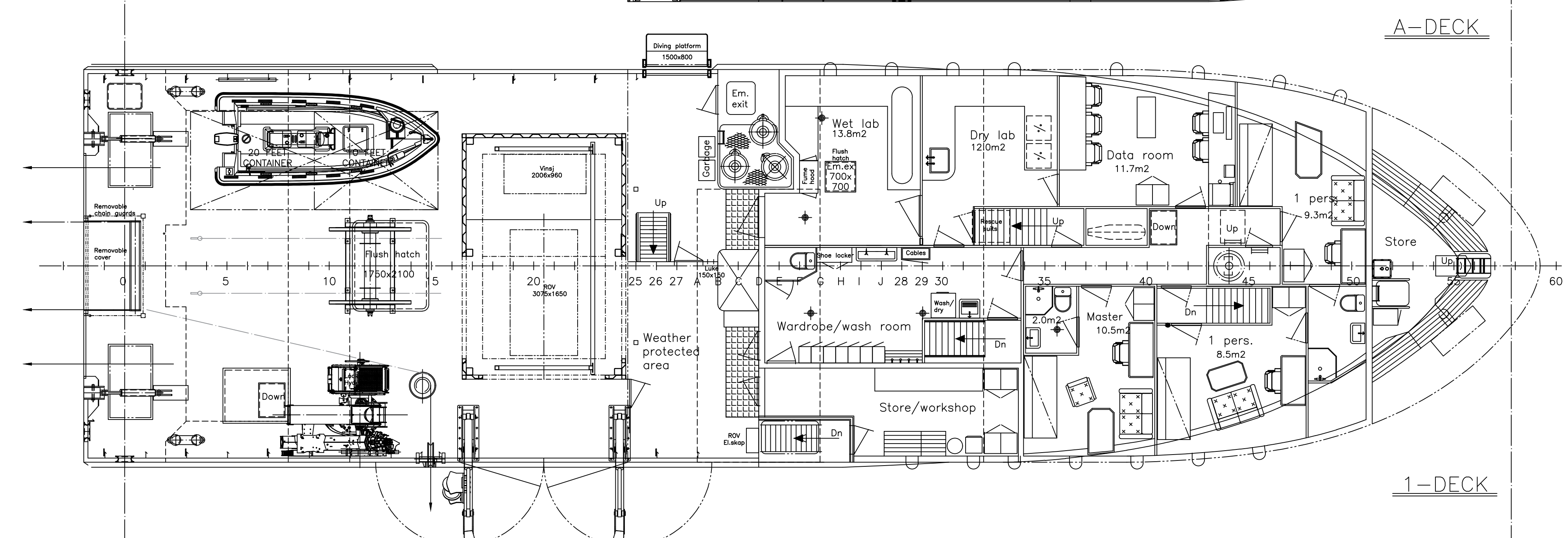
A-DECK
